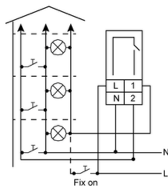
Conexión a 3 hilos 3 wire connection
