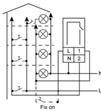
Conexión a 4 hilos 4 wire connection
